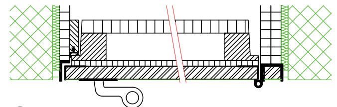
16 RF1 mit Falzdeckel und Alu-Begrenzungswinkel, inkl. Fermacell.
