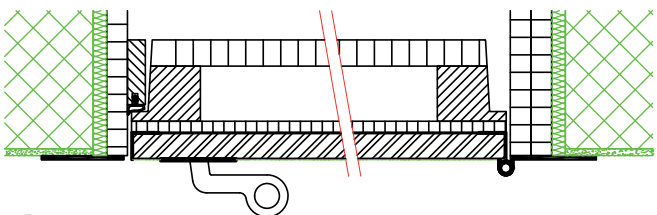
15 RF1/BSP30 mit Flachstahlrahmen auf Futter und Winkeleisenrahmen auf Deckel, inkl. Fermacell
