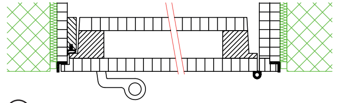
5 Falzdeckel mit Stahl-Begrenzungswinkel auf Futter
