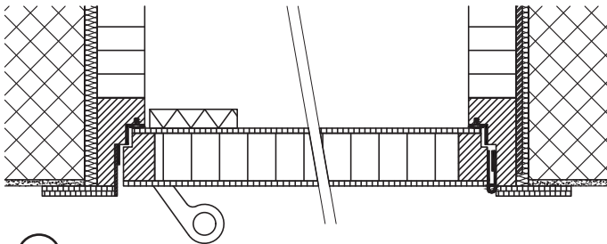
8 HDF Abdeckleiste 60 x 8 mm
