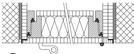
5 mit Falzdeckel und Stahlbegrenzungswinkel auf Futter
