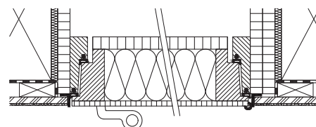
13 Alu-Begrenzungswinkel auf Futter 15 oder 20 mm vorstehend
