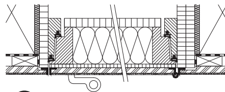
6 für bauseitige Putzträgerplatte mit Alu-Begrenzungswinkel auf Futter und Deckel 15 oder 20 mm vorstehend
