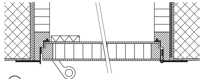
10 Flachstahlrahmen 60 x 3 mm
