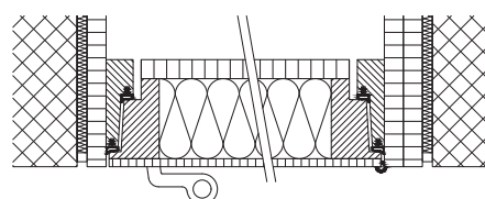
14 mit sichtbarem Futter
