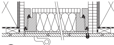
1 für Täfer 13 - 20 mm Täferstärke angeben
