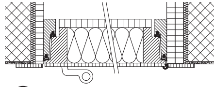
2 MDF Abdeckleiste 60 x 8
