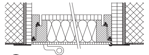
3 Flachstahlrahmen 60 x 3 mm
